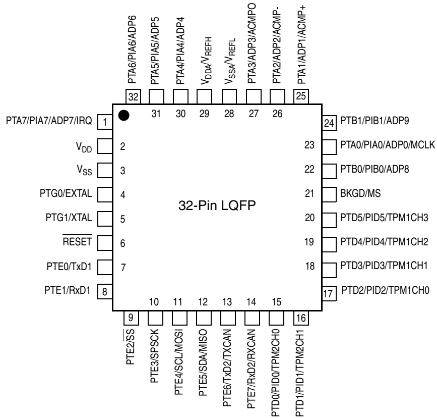
图 2-3. 32 管脚 LQFP
