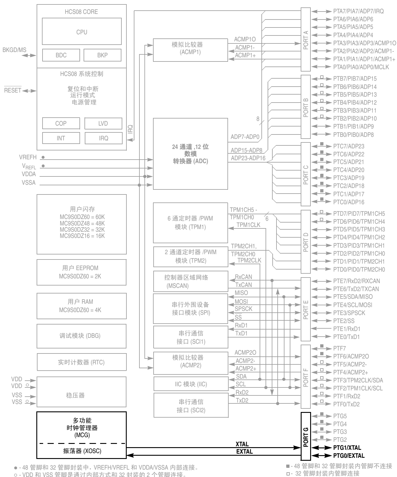
图 8-1. MC9S08DZ60 结构图
