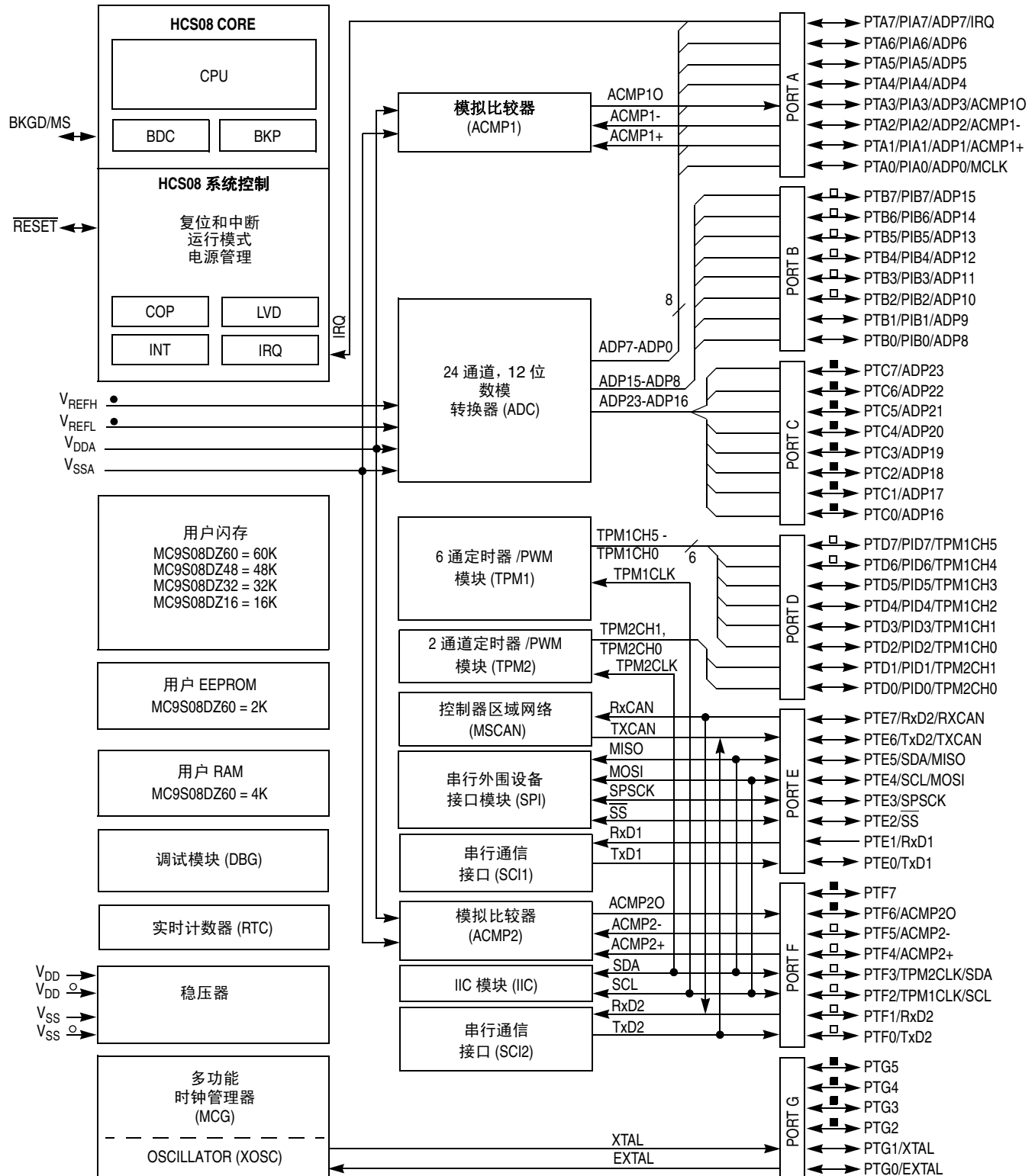
图 1-1. MC9S08DZ60 结构图
