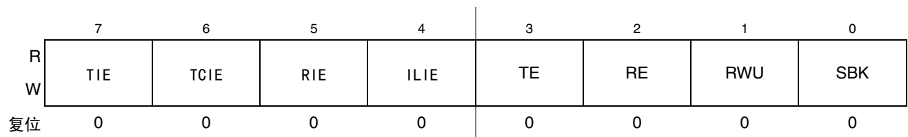
图 14-7. SCI 控制寄存器 2 (SCIxC2)
