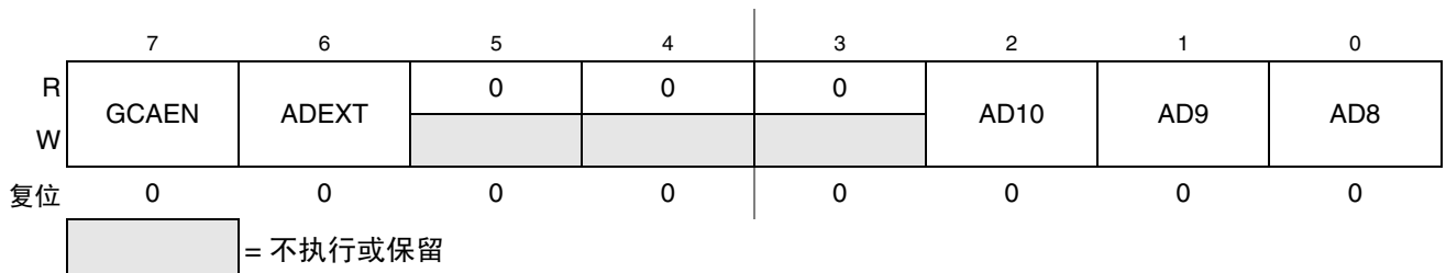
图 11-8. IIC 控制寄存器 (IICC2)
