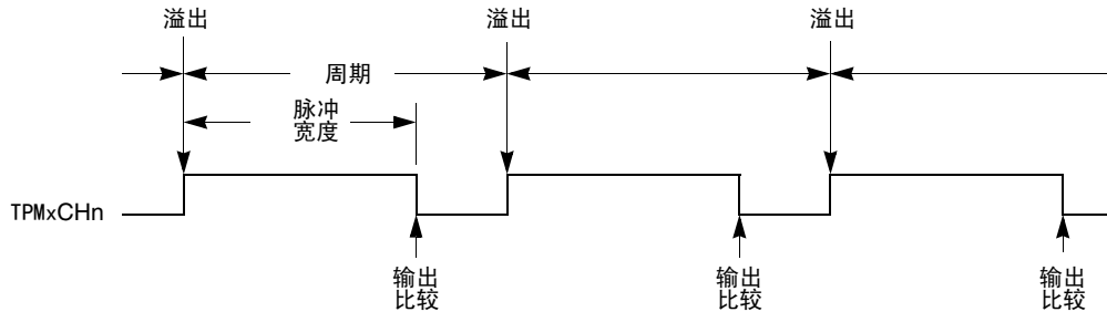
图 16-15. PWM 周期和脉冲宽度 (ELSnA=0)
